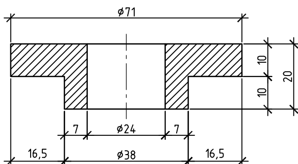
Оправка для запрессовки подшипника в поворотный кулак
