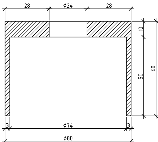
Чашка для выпрессовки и запрессовки
