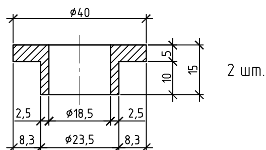
Дистанционные втулки
