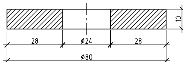
Оправка для запрессовки
