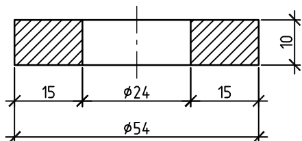
Оправка для запрессовки ступицы в поворотный кулак
